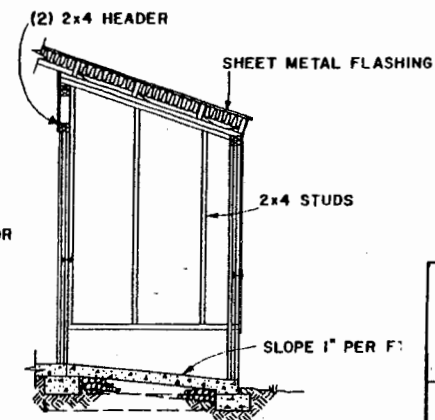
SECTION D-D
