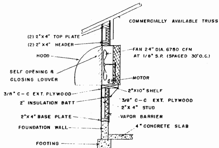
FAN DETAILS
