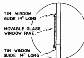
WINDOW SECTION SCALE: 2" = 1'-0"
