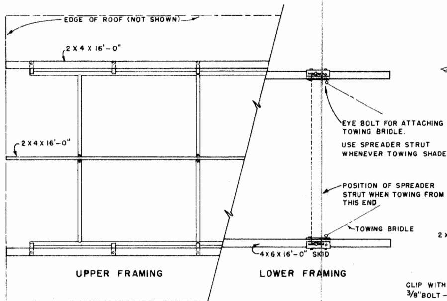
PLAN SCALE: 1/2"=1'-0"
